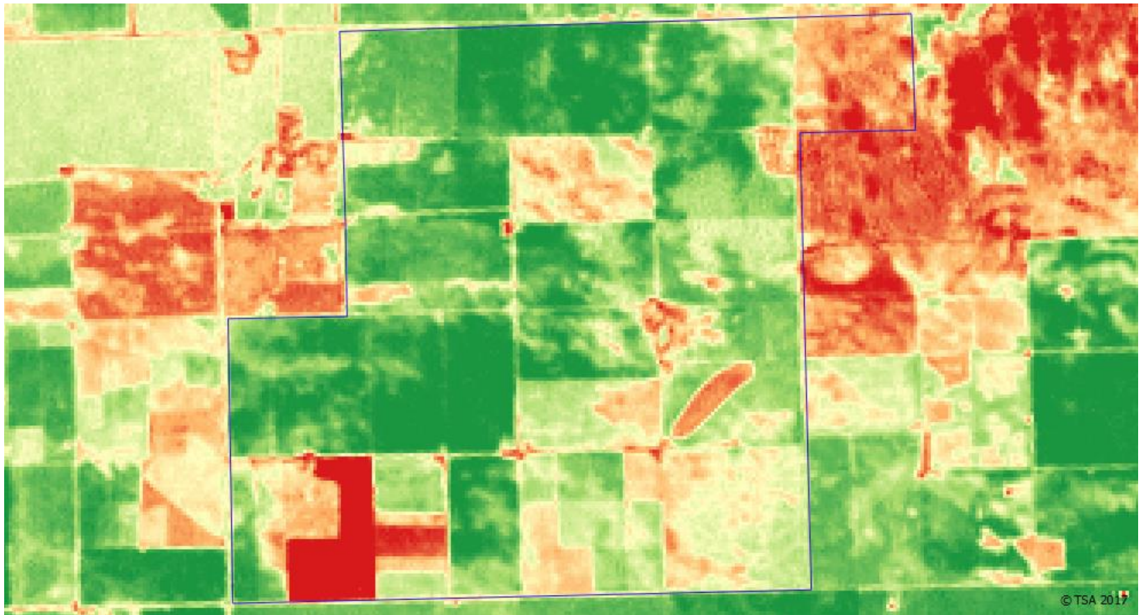
NDVI 14-2-2011
