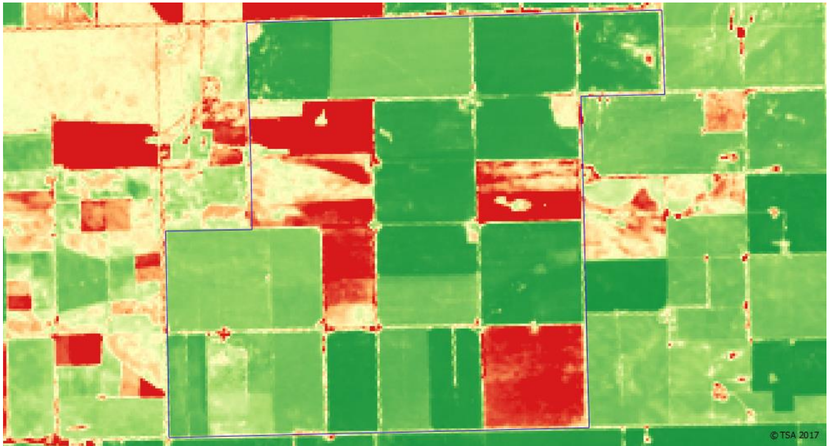
NDVI 4-3-2015
