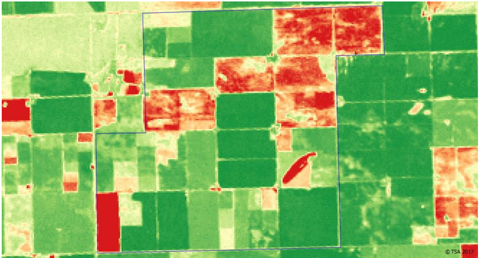
NDVI 1-3-2008
