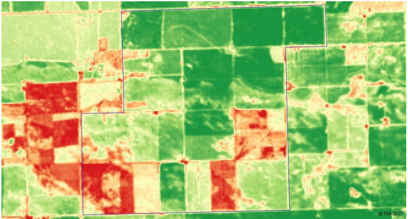
NDVI 3-2-2013
