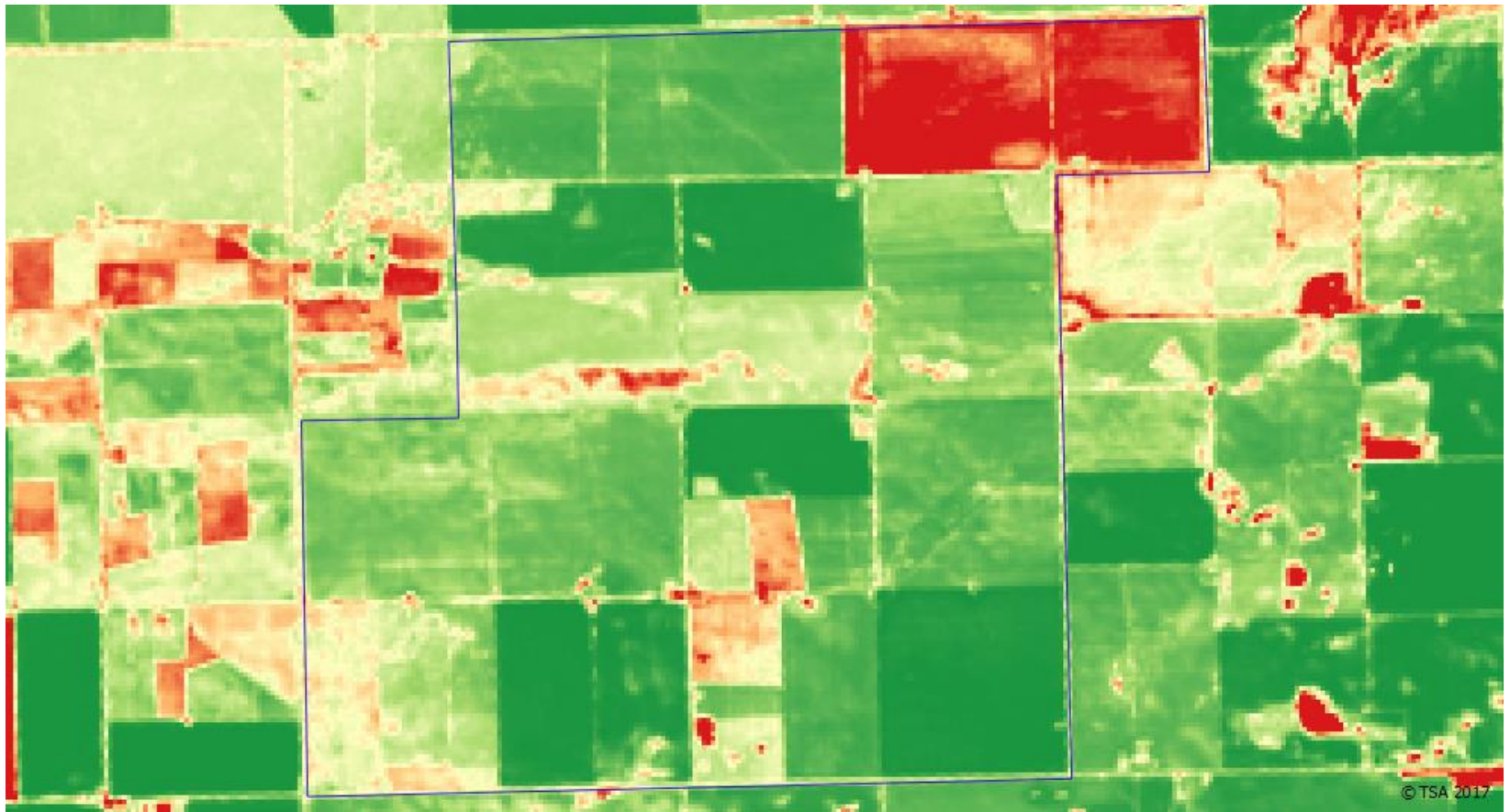
NDVI 6-2-2017
